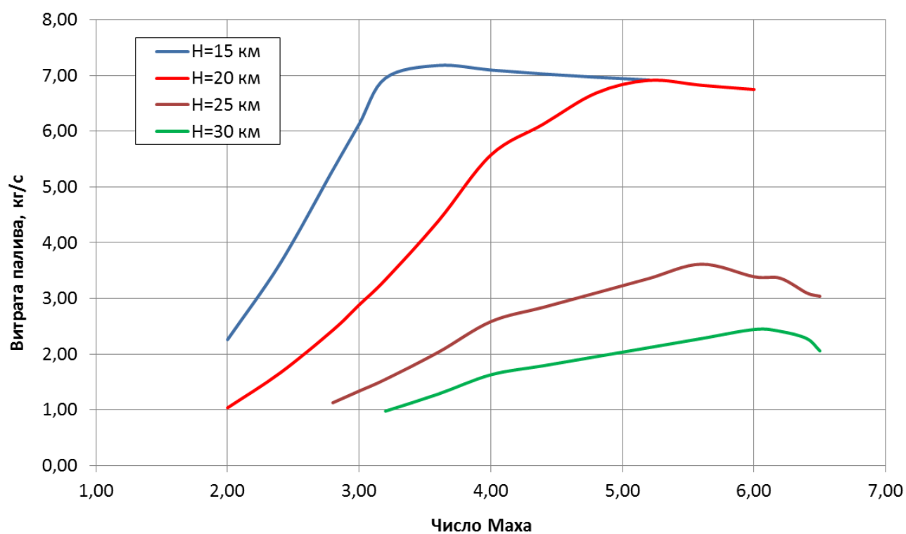
Рисунок 4.13 – Характеристики ППРД
