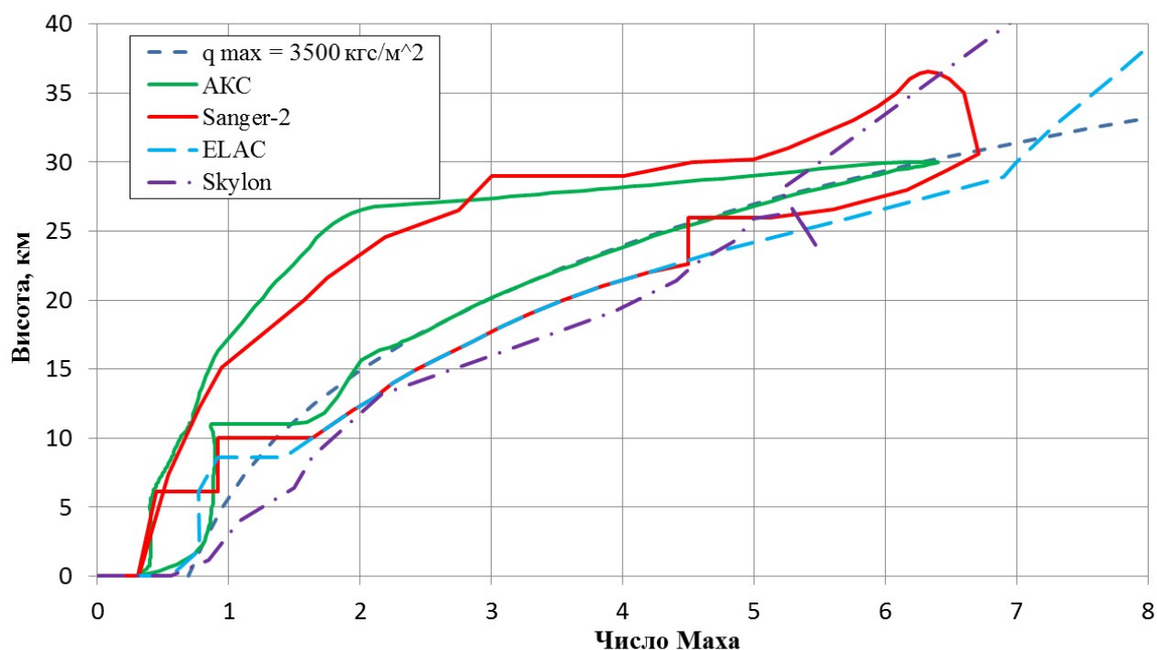
Рисунок 5.5 – Порівняння траєкторій польоту БПЛА
