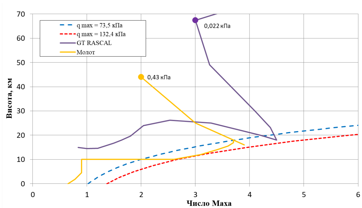
Рисунок 3.2 – Траєкторії польоту та швидкісні напори GT RASCAL та Молот
