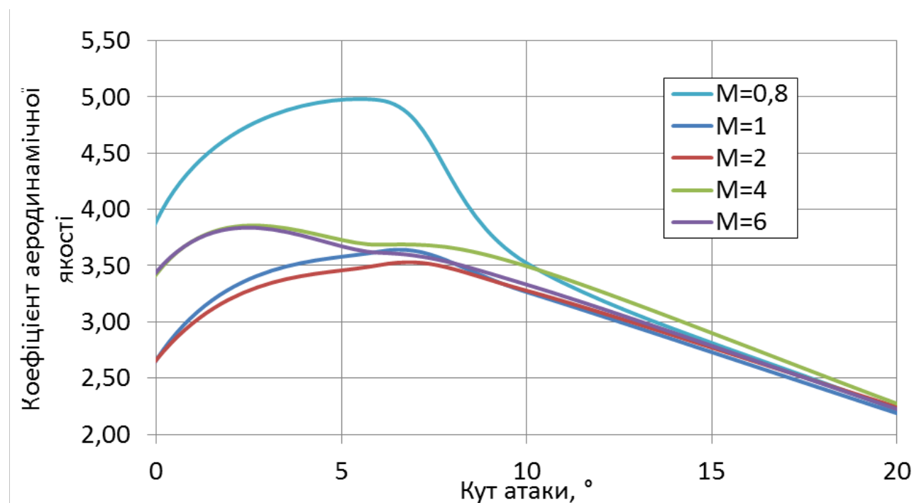
Рисунок 4.17 – Залежність коефіцієнту аеродинамічної якості від кута атаки
