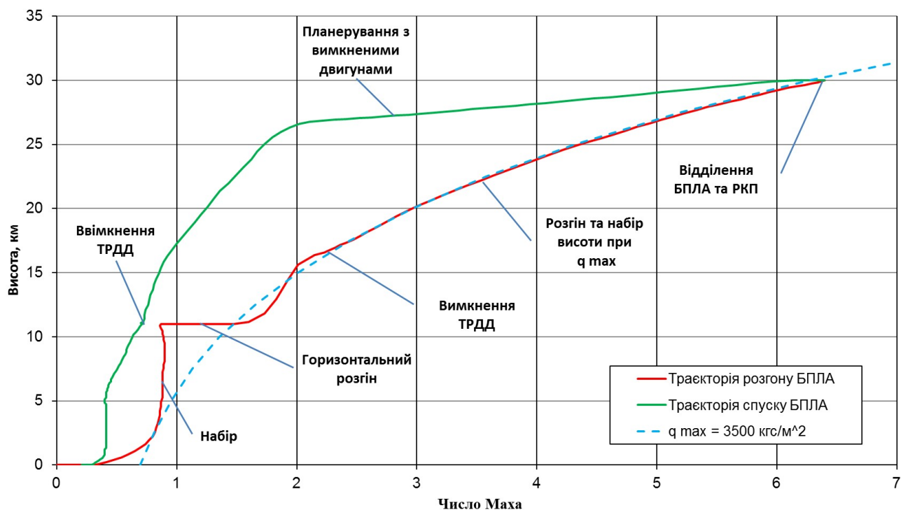
Рисунок 4.20 – Траєкторія польоту РКП (залежність числа Маха від висоти польоту)
