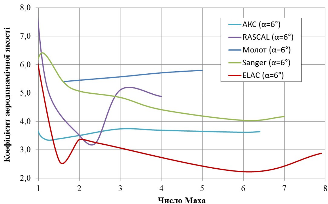
Рисунок 5.3 – Порівняння коефіцієнту аеродинамічної якості при куті атаки 6^\circ
